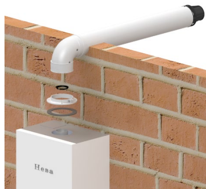
Рис. 3 Схема присоединения коаксиального дымохода Ø 100 / Ø 60 (мм) к котлу
