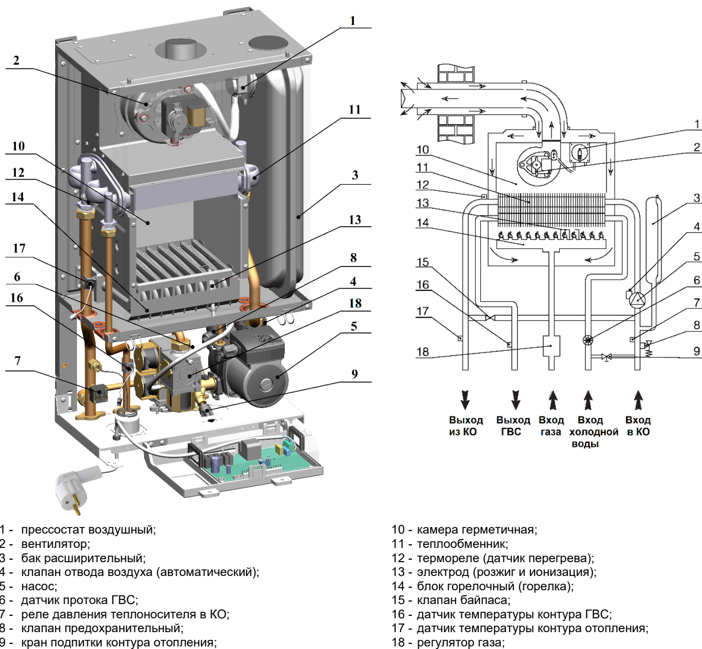
Рис. 7 Функциональная схема котла NEVALUX 7224
